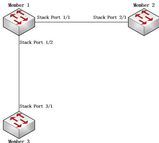
图 10-16 3 台成员设备组成链型拓扑
