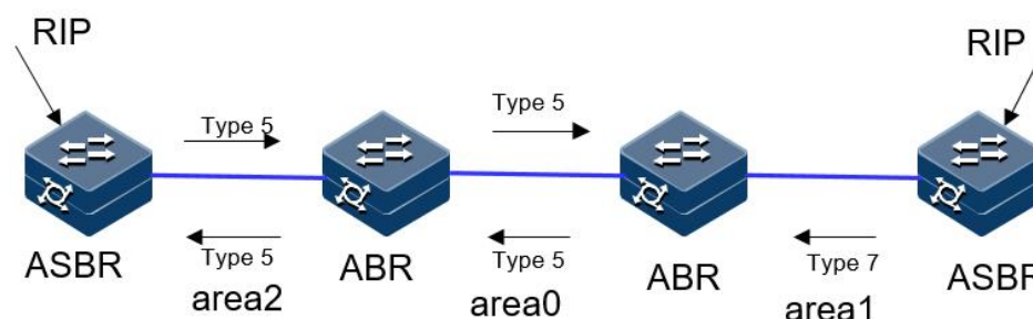
图 3-38 OSPFV3 NSSA 区域示意图
