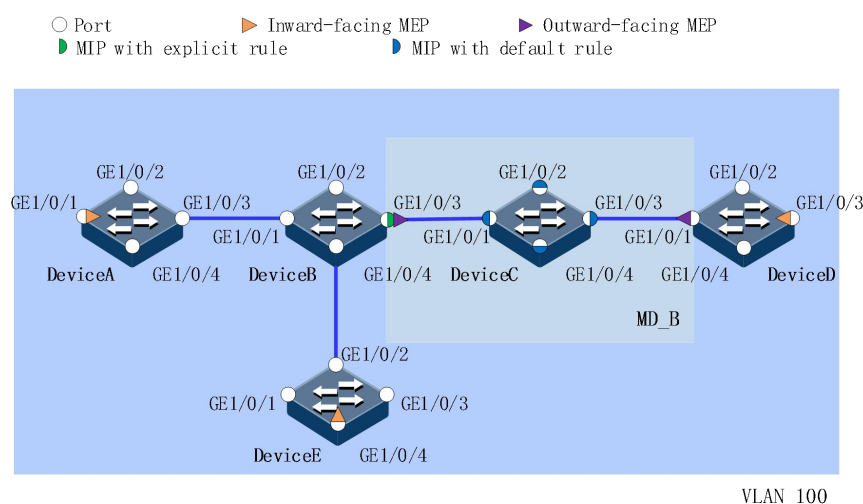
图 7-7 CFM 典型配置组网图
