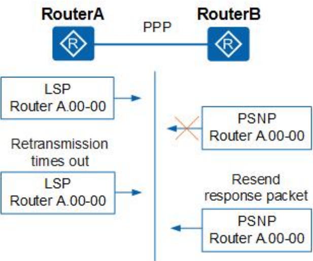
图 3-46 P2P 链路上 LSDB 数据库的同步过程
