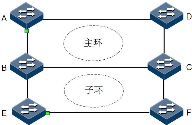
图 9-6 子环模型
